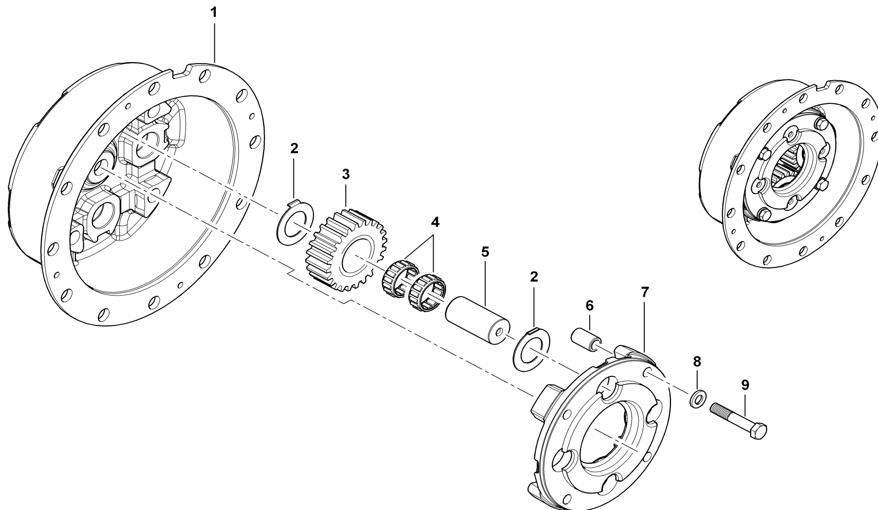
Planetentrieb 2218.013.A
