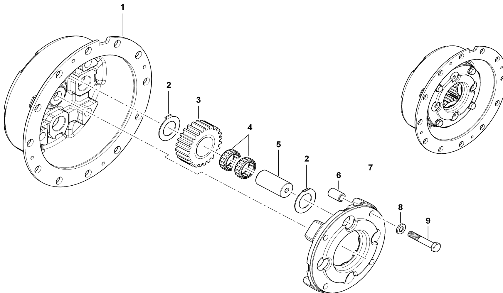
Planetentrieb 2218.013.A
