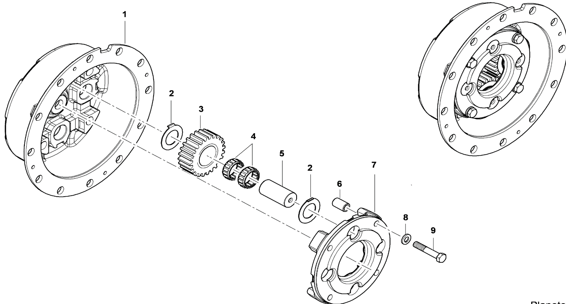
Planetentrieb 2218.033.A
