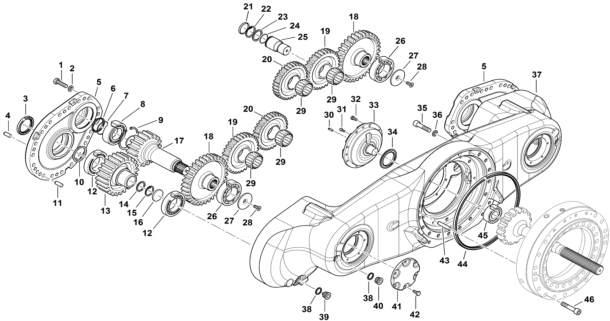
Tandemachsträger 2405.189.A
