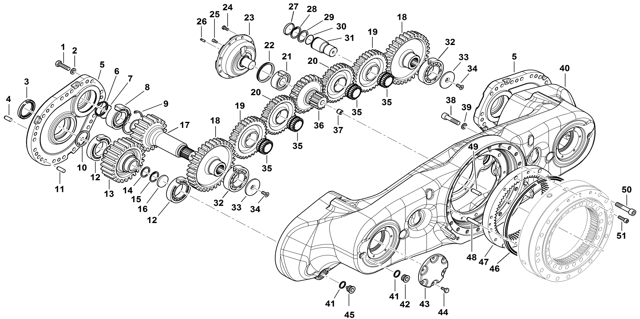
Tandemachsträger 2405.205.A
